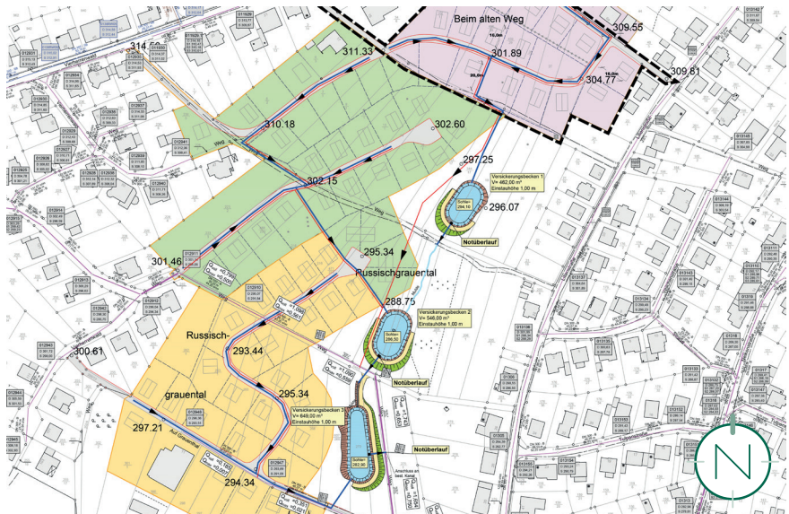
Vorplanung Gesamterschließung 1., 2. und 3. BA, Quelle: PJG GmbH; Stand: Januar 2016
