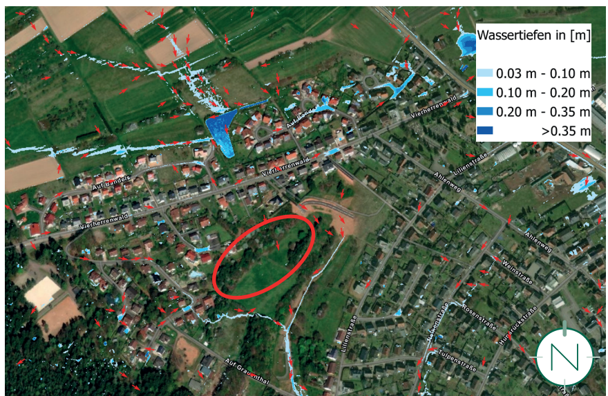
Starkregengefahrenkarte Gemeinde Losheim am See, Quelle: CAD Werkstatt; Stand: 25.05.2022
