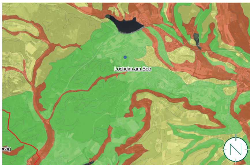
Versickerungsfähigkeit des Bodens (grün = geeignet, gelb = bedingt geeignet, rot = ungeeignet); Quelle: LVGL, GeoPortal Saarland, Stand der Abfrage: 15.10.2024)
